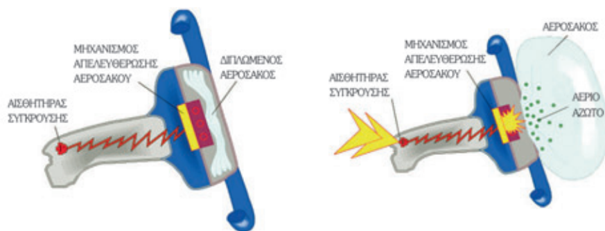
Σχήμα 4.1. Λειτουργία αερόσακου.
